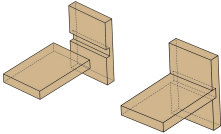
डेडो जोड़
